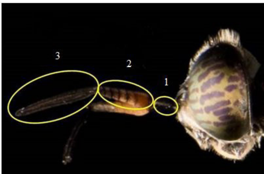
Рис. 3. Строение усиков Hermetia illucens (Jonathan Tan). Круги представляют собой пронумерованные части усиков (1 – скеп, 2 – базальная часть флагеллума, 3 – апикальная часть флагеллума)
