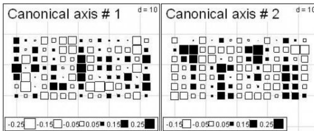
Рис. 4. Пространственное размещение канонических осей широкомасштабных и детальномасштабных компонент
