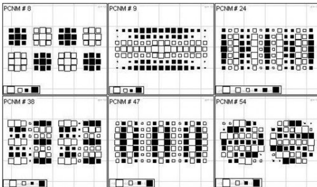
Рис. 3. Пространственное размещение значений PCNM-переменных
