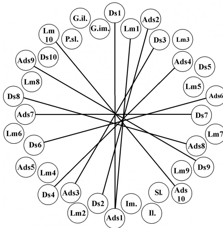
Рис. 2. Коррелограмма величины асимметрии признаков фоллидоза |L - R| . Линиями обозначены сильно коррелирующие признаки ( p < 0.05 ) Fig. 2. Correlogram of the asymmetry of the foliosis signs |L - R| . The lines indicate strongly correlating traits ( p < 0.05 )
