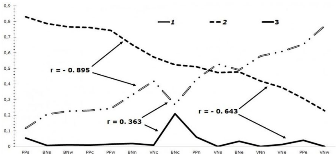
Рис. 3. Зависимость встречаемости синантропных гекконов, совместно обитающих на территории городов. D - индекс доминирования; BN - Бангкок; PP - Пномпень; VN - Вьентьян; с - центр города; n - северная окраина; s - южная окраина; w - западная окраина; e - восточная окраина, 1 - H. frenatus , 2 - H. platyurus , 3 - другие виды
