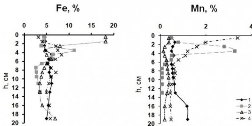
Рис. 5. Вертикальное распределение Fe и Mn в поверхностном слое ДО центрального района Онежского озера. 1 – глубина залегания 42 м, 2 – 48 м, 3 – 81 м, 4 – 85 м Fig. 5. Vertical distribution of Fe and Mn in the surface layer of bottom sediments of the central region of Lake Onega: 1 – depth of occurrence 42 м, 2 – 48 м, 3 – 81 м, 4 – 85 м
