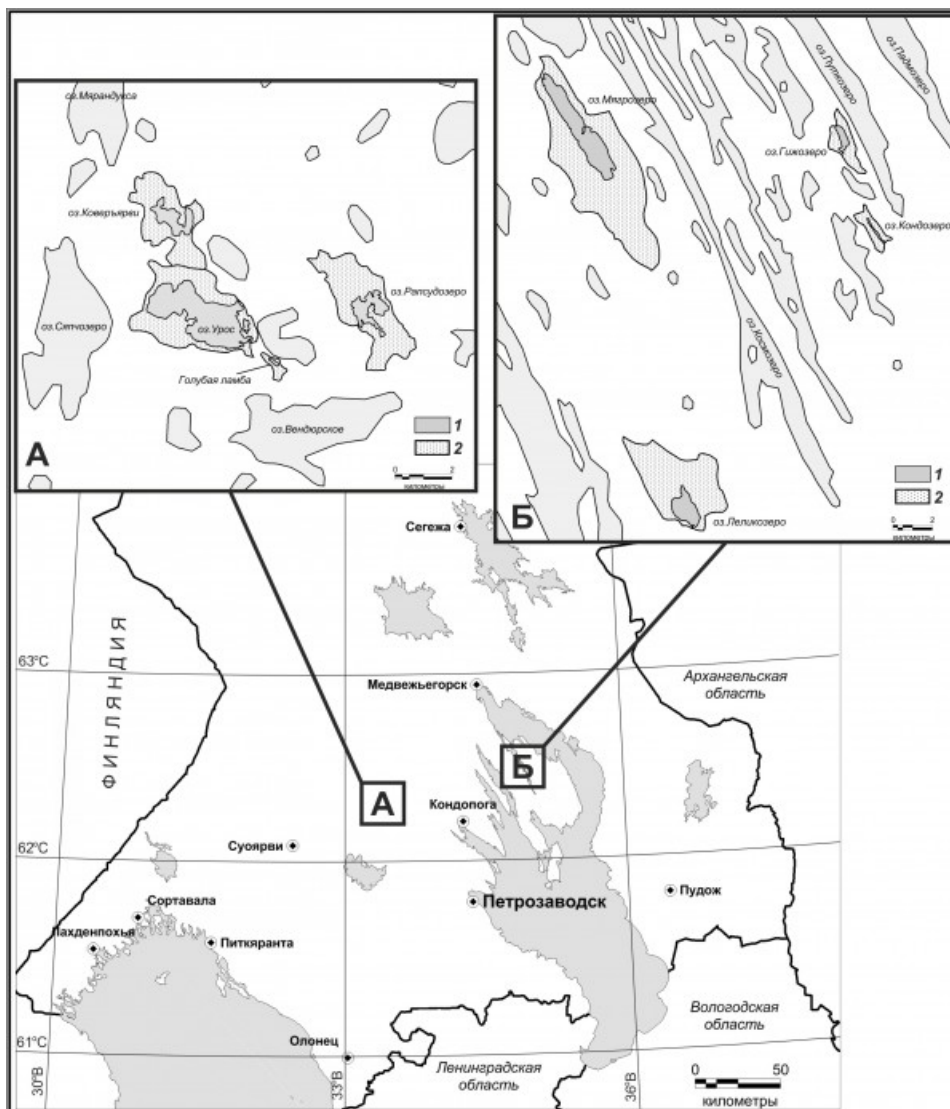
Рис. 1. Карта-схема расположения озер: А – Вохтозерская ледораздельная возвышенность; Б – Заонежский полуостров; 1 – озеро; 2 – водосборная территория Fig. 1. Scheme of the location of studied lakes: A – Vohtozerskaya iceshed height; Б –
