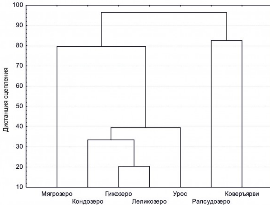
Рис. 2. Дендрограмма классификации изученных озер методом ближайшего соседа. Одиночное сцепление
