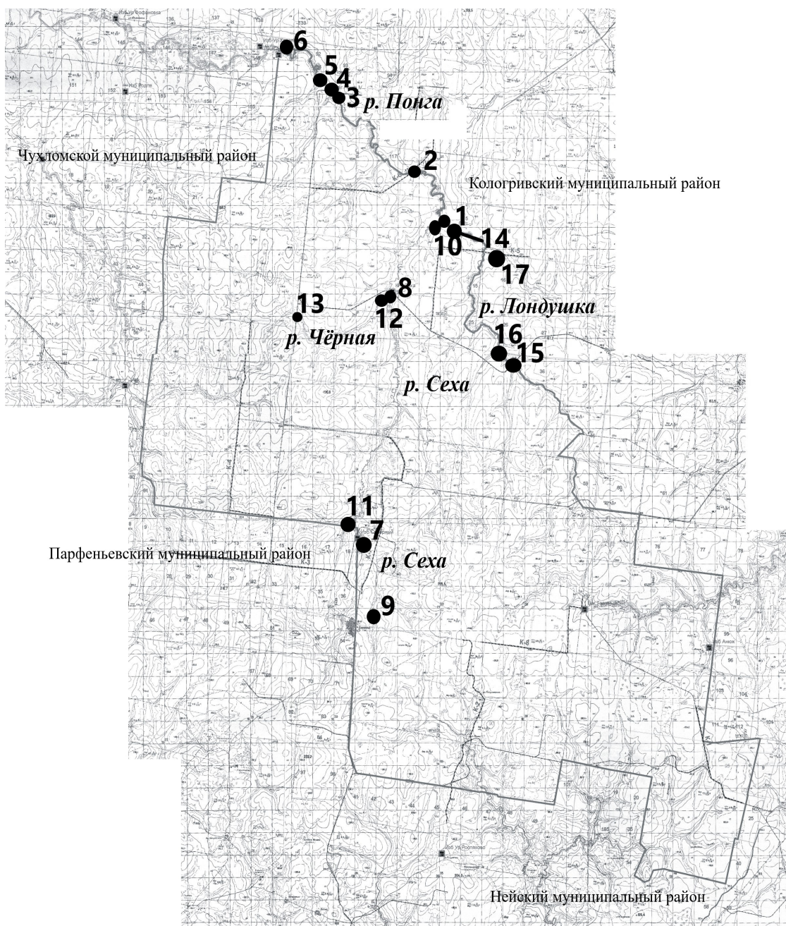
Рис. 1. Карта-схема расположения станций отбора проб зообентоса на территории кологривского кластера заповедника р. Понга: 1, 2 – верхнее течение; 3 – среднее течение, бобровый пруд; 4, 5, 6 – среднее течение; р. Сеха: 7, 9 – верхнее течение; 8 – среднее течение; 10 – нижнее течение; 11 – бобровый пруд; р. Чёрная: 12 – нижнее течение; 13 – среднее течение; р. Лондушка – 14 нижнее течение; 15 – среднее течение; 16 – бобровый пруд р. Ломенга – 17.
