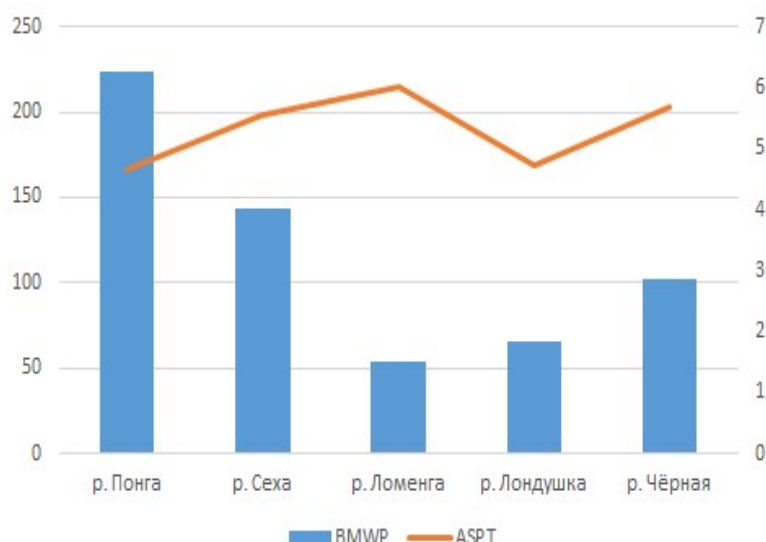
Рис. 5. Значение индексов BMWP и ASPT исследованных рек заповедника Fig. 5. The value of the BMWP and ASPT indices of the studied rivers of the reserve
