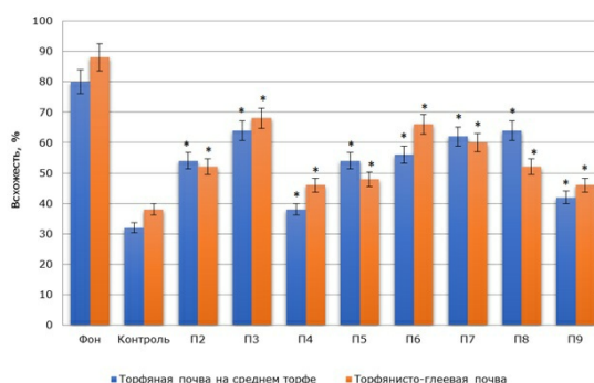
Рис. 2. Результаты оценки всхожести семян в исследуемых образцах.
