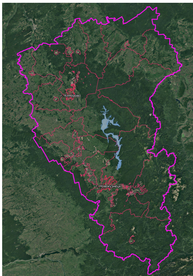
Рис. 1. Плановые границы Крапивинского водохранилища в случае его достройки Fig. 1. Planned boundaries of the Krapivinsky reservoir in case of its completion
