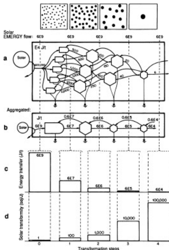
Рис. 2. Иерархия энергий: а – сеть с энергетическими потоками, б – преобразованная энергетическая сеть в цепь, с – график энергетических потоков на каждом уровне энергетической иерархии, d – солнечные трансформации на каждом уровне иерархии
