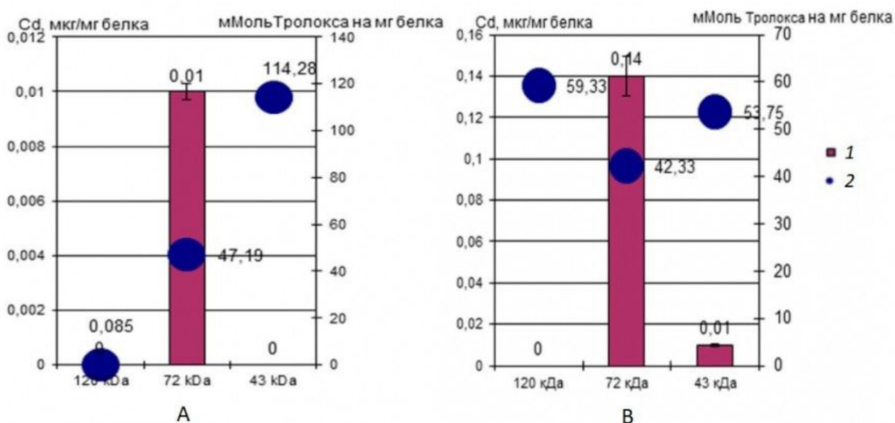
Рис. 7. АО активность (мМоль Тролокса/мг белка) среди МТ-подобных белков пищеварительной железы двухлетних особей приморского гребешка M. yessoensis контрольной (А) и экспериментальной групп ( CdCl_2 , 300 мкг/л) (В)
