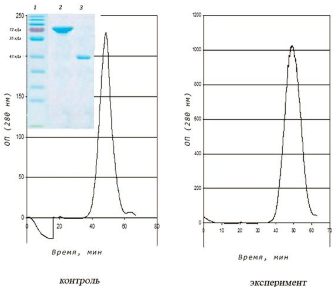
Рис. 8. Хроматографический профиль (FPLC, Superosa 12, \lambda 280 нм) ресуспандированного ацетонного осадка пищеварительной железы трехлетних особей приморского гребешка M. yessoensis (контроль и эксперимент – \text{CdCl}_2 300 мкг/л)
