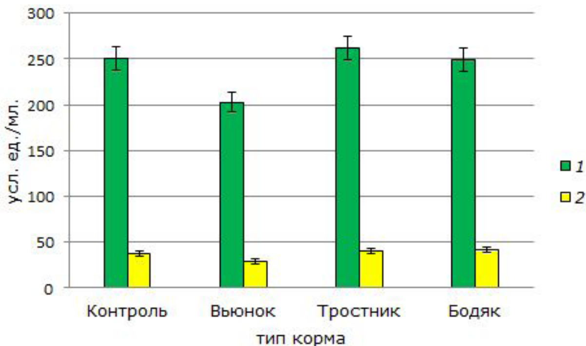
Рис. 3. Влияние дополнительных растительных компонентов в составе сочных кормов на активность антиоксидантных ферментов в плазме крови кролика: 1 – супероксиддисмутаза, 2 – каталаза
