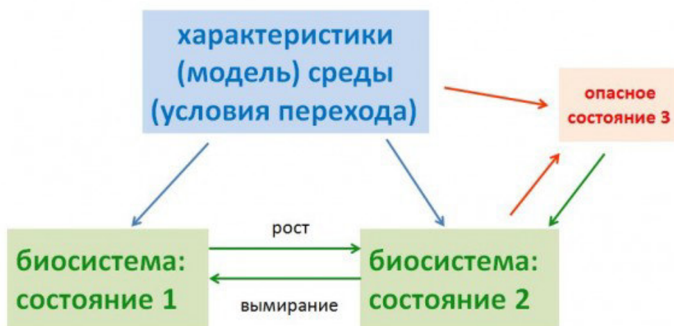
Рис. 3. Простейшая модель биосистемы в виде конечного автомата Fig. 3. Simplest model of biosistem as a finite state machine
