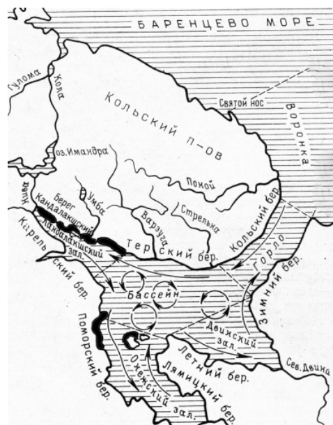
Рис. 1. Картограмма Белого моря (Наумов, Оленев, 1981). Стрелками показана циркуляция вод, черными полосами - места сбора материалов Fig. 1. Schematic map of the White Sea (Naumov, Olenev, 1981). The arrows indicate the water circulation, black stripes - places of material collection
