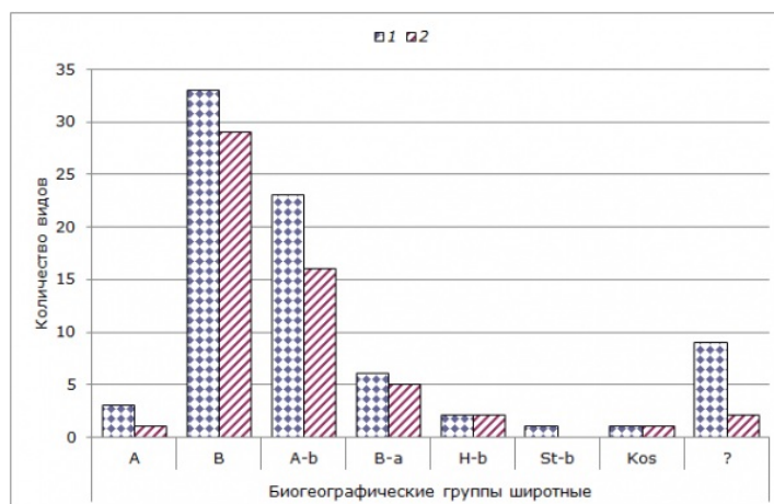
Рис. 5. Распределение биохорологических (по общности биоэкологических адаптивных связей) групп беспозвоночных на литорали Кандалакшского (1) и Онежского (2) заливов. По оси ординат – количество видов
