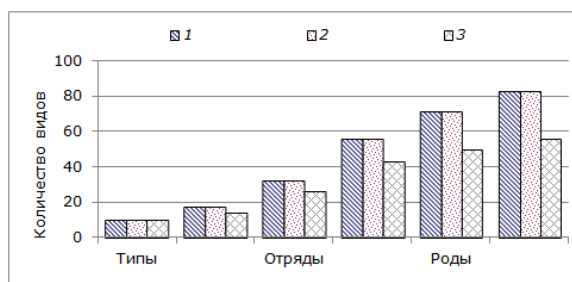
Рис. 2. Таксономическая представленность морских беспозвоночных на литорали всей исследованной акватории (1), Кандалакшского (2) и Онежского (3) заливов Белого моря
