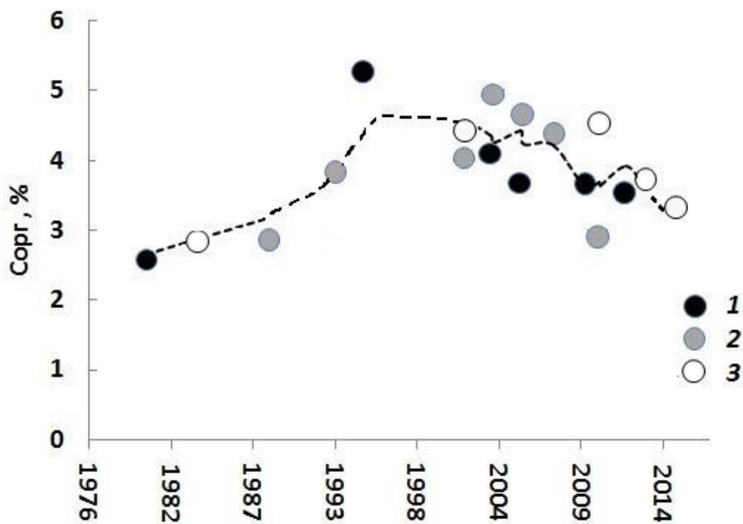
Рис. 4. Динамика изменения концентрации C_{орг} в поверхностном слое (0–5 см) ДО; ст. C1; 1 – июнь, 2 – август, 3 – сентябрь
