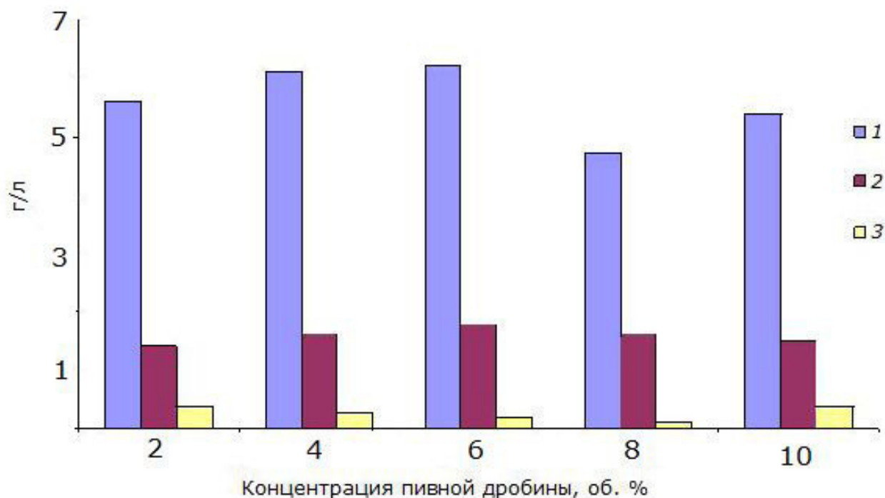
Рис. 1. Выход целевых продуктов в зависимости от концентрации пивной дробины влажностью 82–86 % в сбраживаемой среде: 1 – бутанол, 2 – ацетон, 3 – этанол
