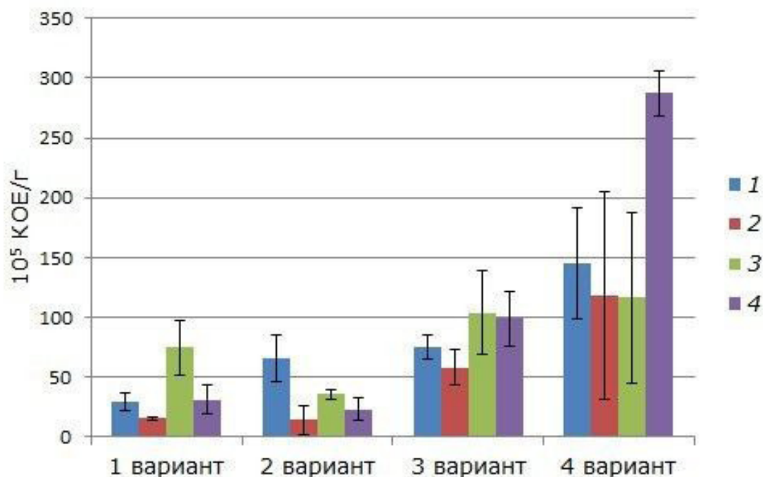
Рис. 2. Численность аммонификаторов и амилотических микроорганизмов через 3.5 месяца после начала проведения модельного опыта по переувлажнению (среднее и стандартные отклонения): 1 – численность аммонификаторов в аллювиальной почве, 2 – численность амилотических микроорганизмов в аллювиальной почве, 3 – численность аммонификаторов в черноземе, 4 – численность амилотических микроорганизмов в черноземе
