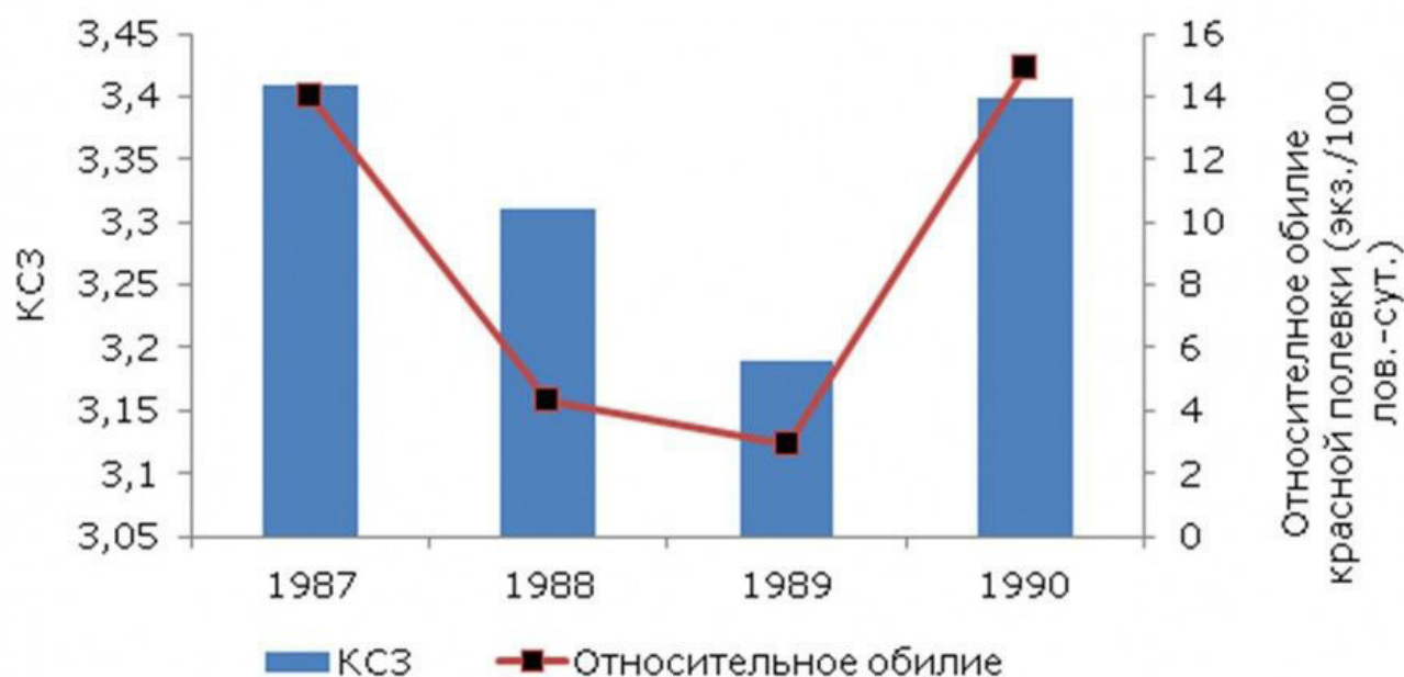
Рис. 3. Зависимость КСЗ МЗ от относительного обилия красной полевки Среднего Приобья Fig. 3. The dependence of the complexity factor of the M3 tooth on the relative abundance of the red vole in the Middle Ob area
