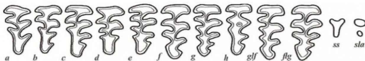
Рис. 2. Вариации рисунка жевательной поверхности зуба М³
