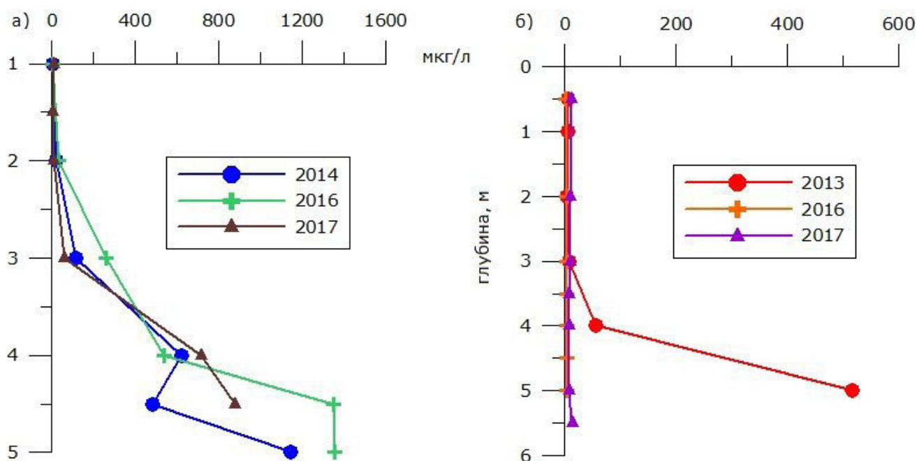
Рис. 3. Распределение сероводорода и сульфидов в водной толще оз. Назаровское а) в зимний и б) летний периоды Fig. 3. Distribution of hydrogen sulfide and sulphides in the water column of Lake Nazarovskoe a) winter and b) summer periods
