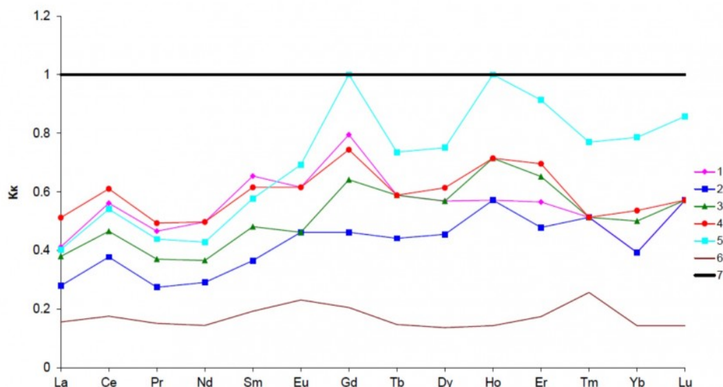
Рис. 2. Кларки концентрации РЗЭ в шунгитовых почвах неразрабатываемых выходов шунгитовых пород Подсосонье (1), Лебещина (2) и Карнаволоок (3) и карьеров Захогино (4) и Максово (5); 6 – фоновые образцы почв; 7 – кларк в почвах мира (Водяницкий, 2009)
