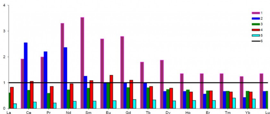
Рис. 4. Коэффициенты обогащения почв РЗЭ относительно подстилающих шунгитовых пород для неразрабатываемых выходов шунгитовых пород Подсосонья (1), Лебещина (2) и Карнаволока (3) и карьеров Захогино (4) и Максово (5). 6 - КОП = 1 (соотношение суммарного валового содержания ( \Sigma REE) в почве и породе равно единице)
