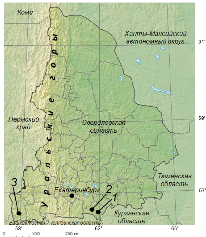
Картосхема Свердловской области с указанием местообитаний прыткой ящерицы Lacerta agilis : 1 – зона многоэтажной застройки г. Каменска-Уральского, 2 –
