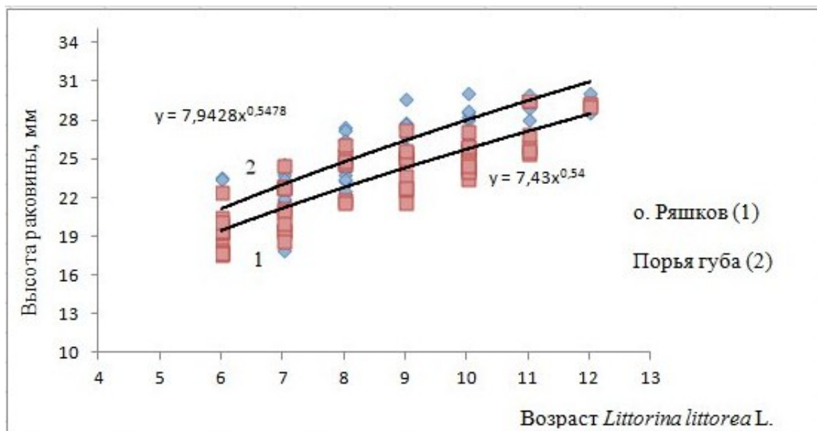
Рис. 3. Модели, описывающие зависимость высоты раковины от возраста моллюска: y = 7.43x^{0.54} для моллюсков с о. Ряшков (1), y = 7.9428x^{0.5478} для моллюсков Порьей губы (2) Fig. 3. Models describing the dependence of the height of shell on its age: y = 7.43x^{0.54} for Littorina littorea from the island Ryachkov (1), y = 7.9428x^{0.5478} for mollusks from the Porya Bay (2)
