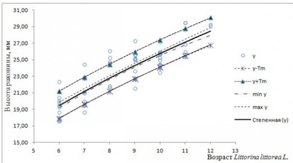
Рис. 4. Линия регрессии ( y ), ее доверительный интервал ( \min y ; \max y ) и интервал прогноза ( y-Tm ; y+Tm ) для модели y_i = 7.43x0.54 (о. Ряшков)
